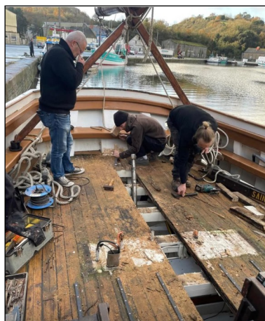
Démontage de l'étambrai ...
